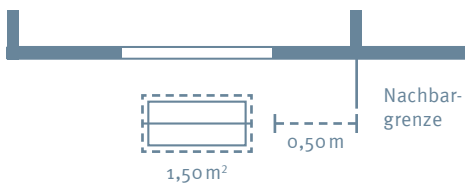
Aufsicht Ladenfront
